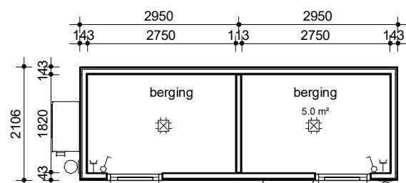
Begane grond
