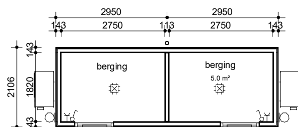
Begane grond
