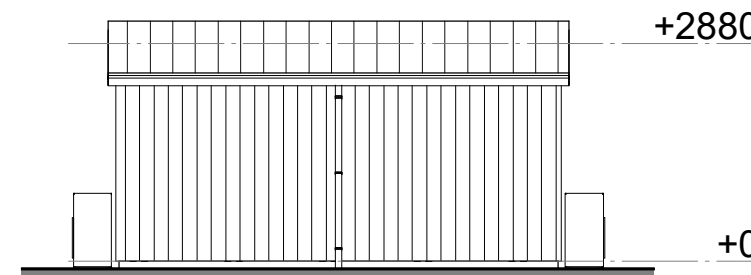
Achtergevel
