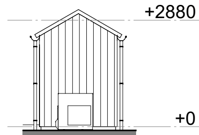
Rechtergevel
