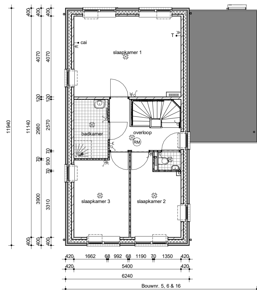
Eerste verdieping
