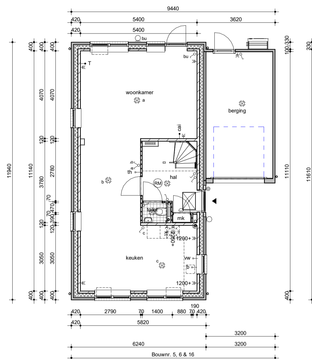
Begane grond
