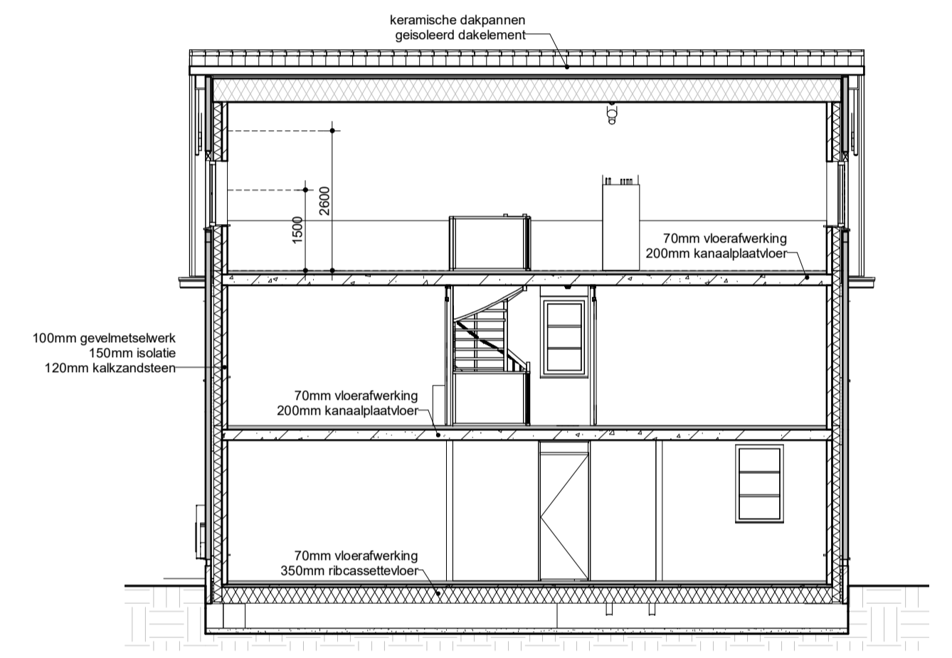
Doorsnede A
