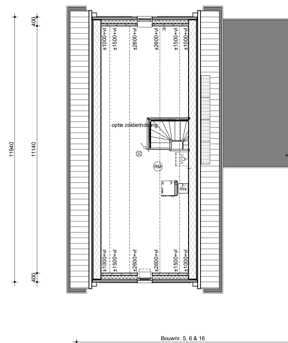
Tweede verdieping
