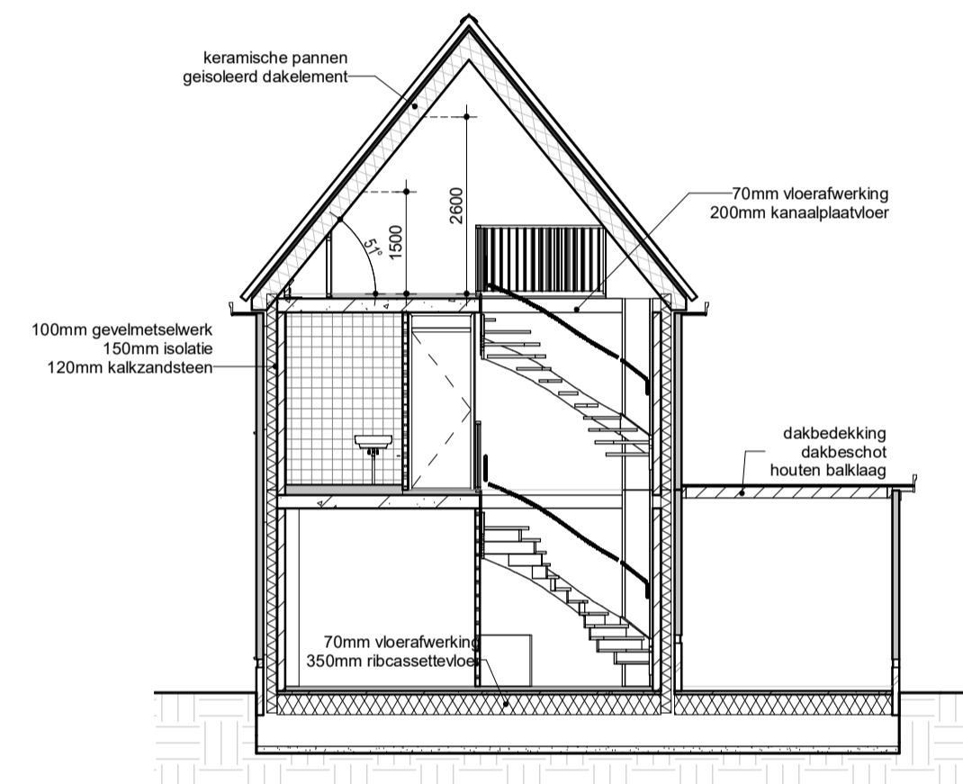
Doorsnede B
