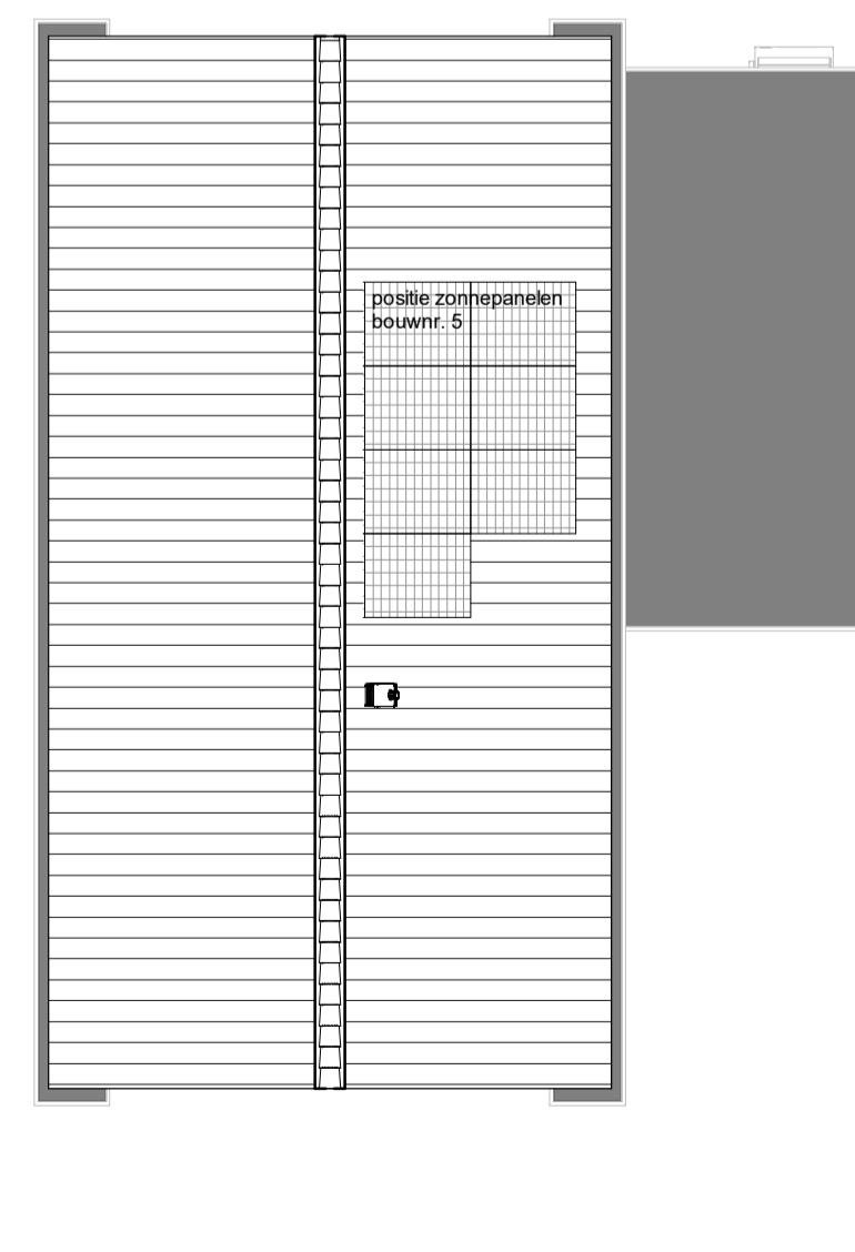
Dakaanzicht bnr. 5
